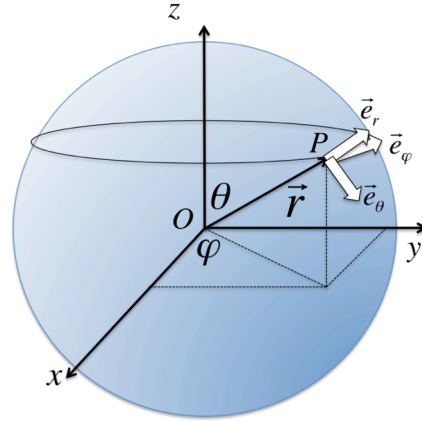
図 9.2 3次元極座標
