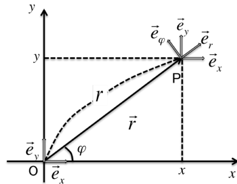
図 9.1 2次元極座標
