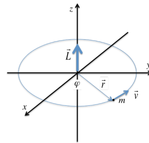
図 10.4 中心力
