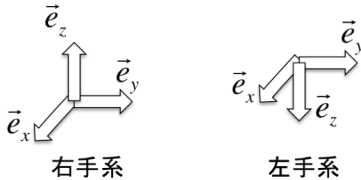
図 10.2
