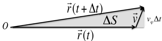
図 10.5 面積速度
