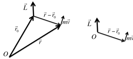
図 10.3 角運動量
