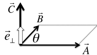
図 10.1 ベクトル積
